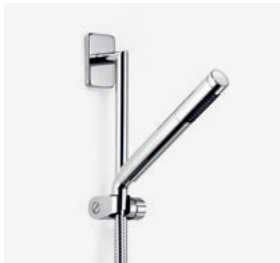
26 402 710 Complete shower set Gruppo doccetta con flessibile e asta saliscendi Juego de ducha de mano con barra corredera [14 l/min.]
