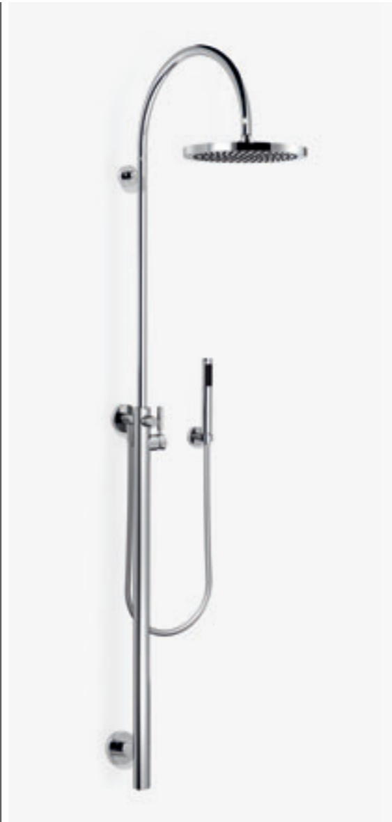
26 023 885* / 26 022 885* Shower system with wall-mounted single-lever shower mixer with/without shower set, Ø 300 mm / Doccia a stelo con miscelatore monocomando doccia esterno con/senza doccia, Ø 300 mm / Teléfono de ducha con batería monomando de ducha para montaje a pared con/sin ducha de mano, Ø 300 mm [14 l/min.]
